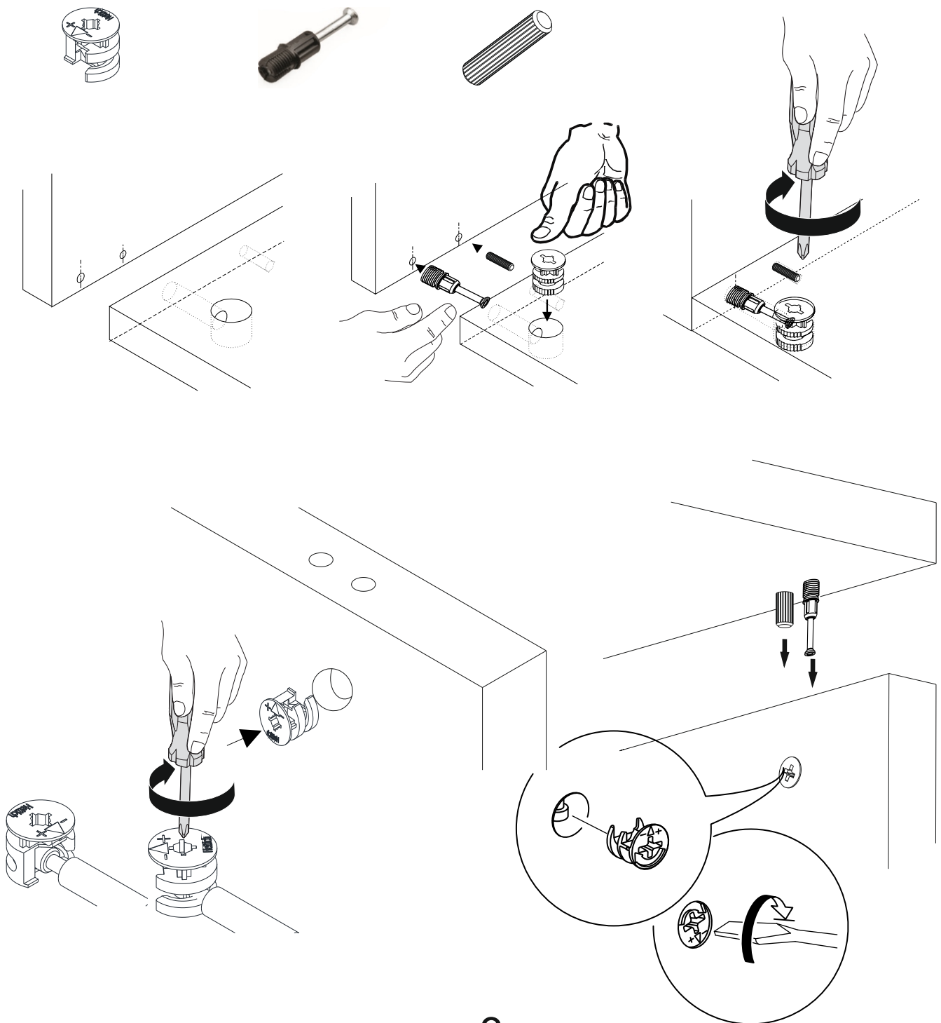
Minifix
